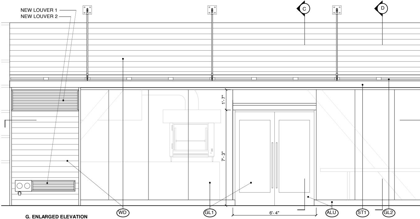
G. ENLARGED ELEVATION
