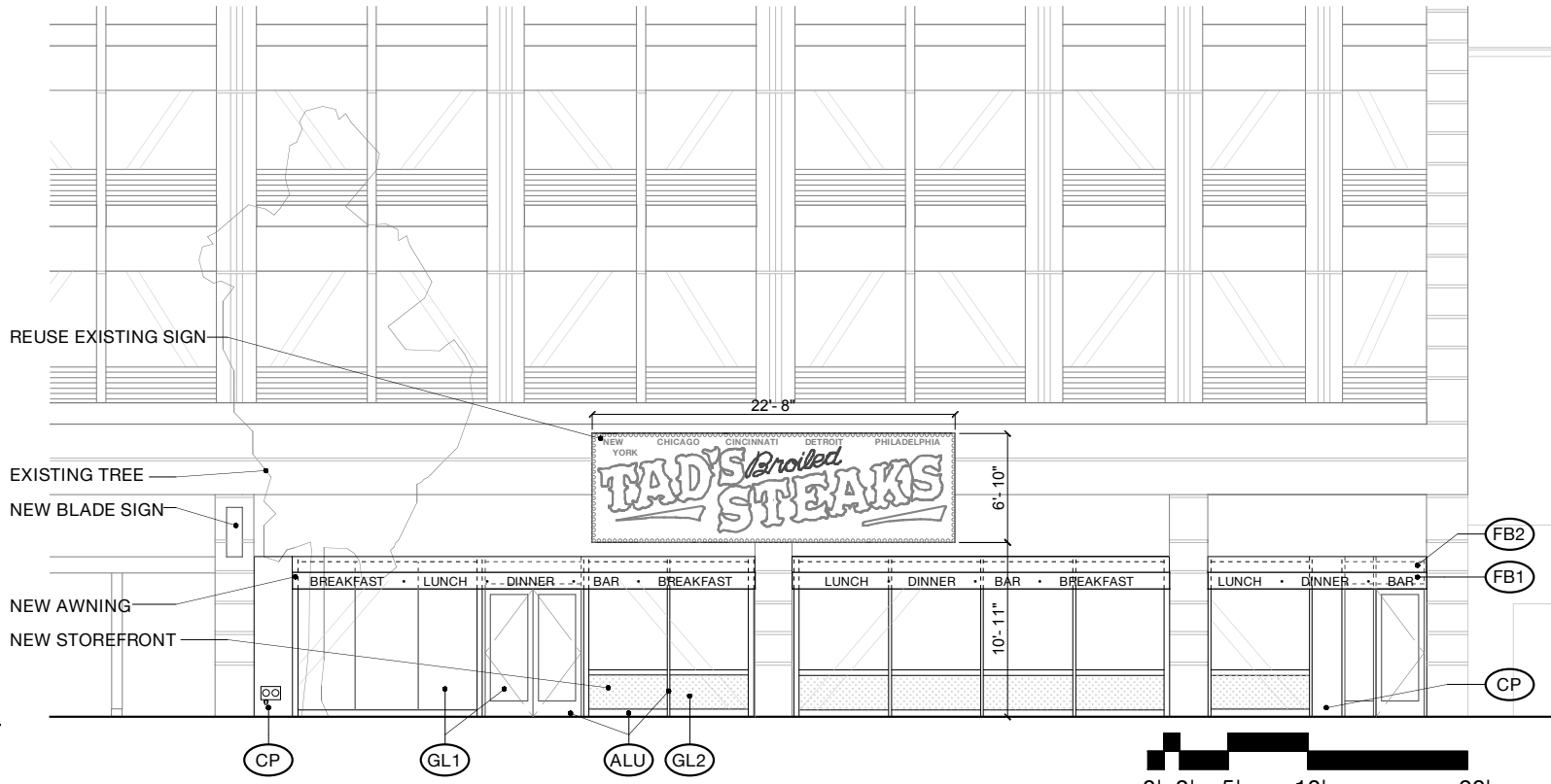
A. EXTERIOR ELEVATION
