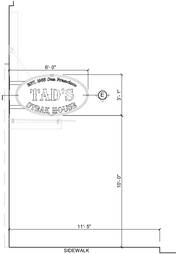
F. BLADE SIGN ELEVATION
