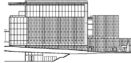
WEST ELEVATION 03 SCALE: 1/8" = 1'-0"
