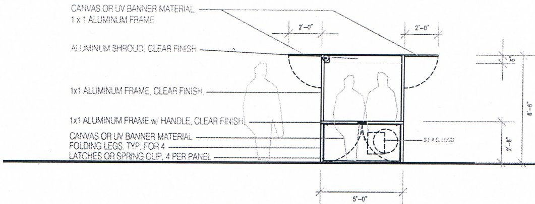
LONG ELEVATION
