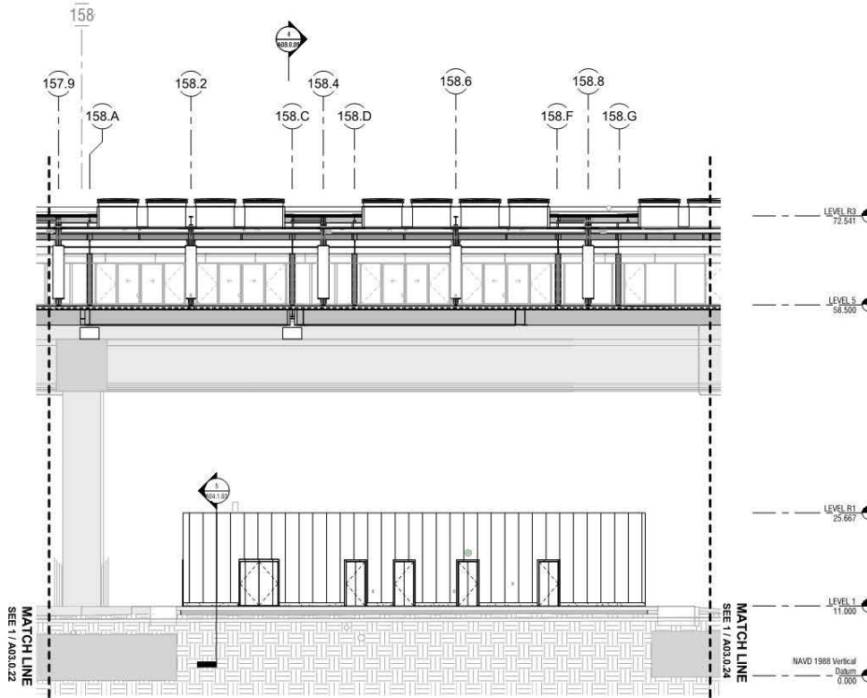
1 LONGITUDINAL SECTION - CENTERLINE SECTOR 2 OF 3 A03.0.21 A03.0.23 SCALE: 1/8" = 1'-0"
