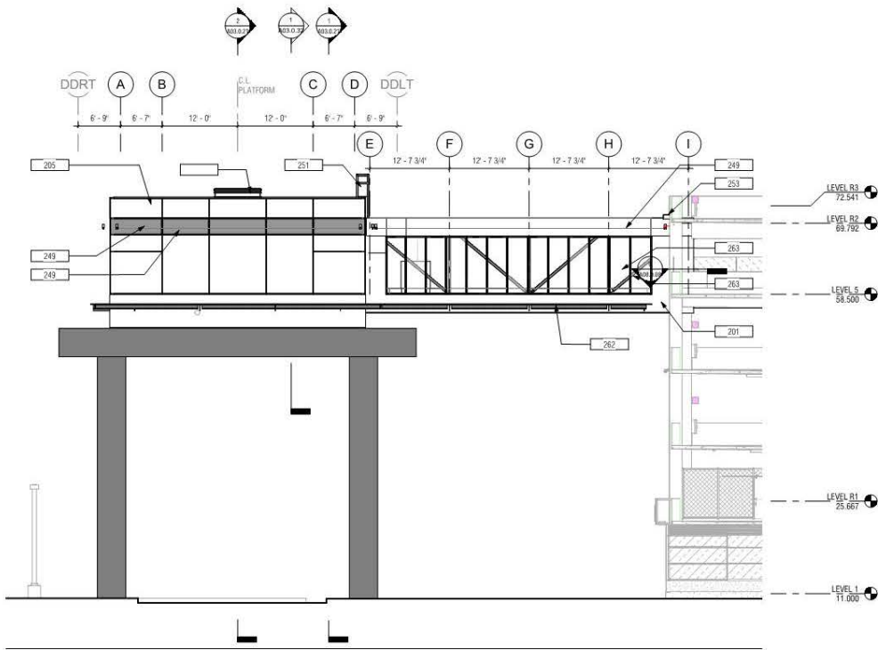
1 EXTERIOR ELEVATION - NORTH A03.0.08 SCALE: 1/8" = 1'-0"
