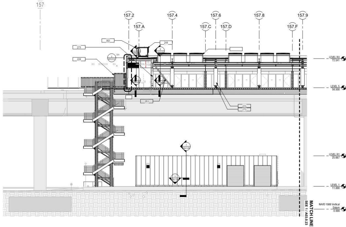
1 LONGITUDINAL SECTION - CENTERLINE SECTOR 1 OF 3 A03.0.21 A03.0.22 SCALE: 1/8" = 1'-0"
