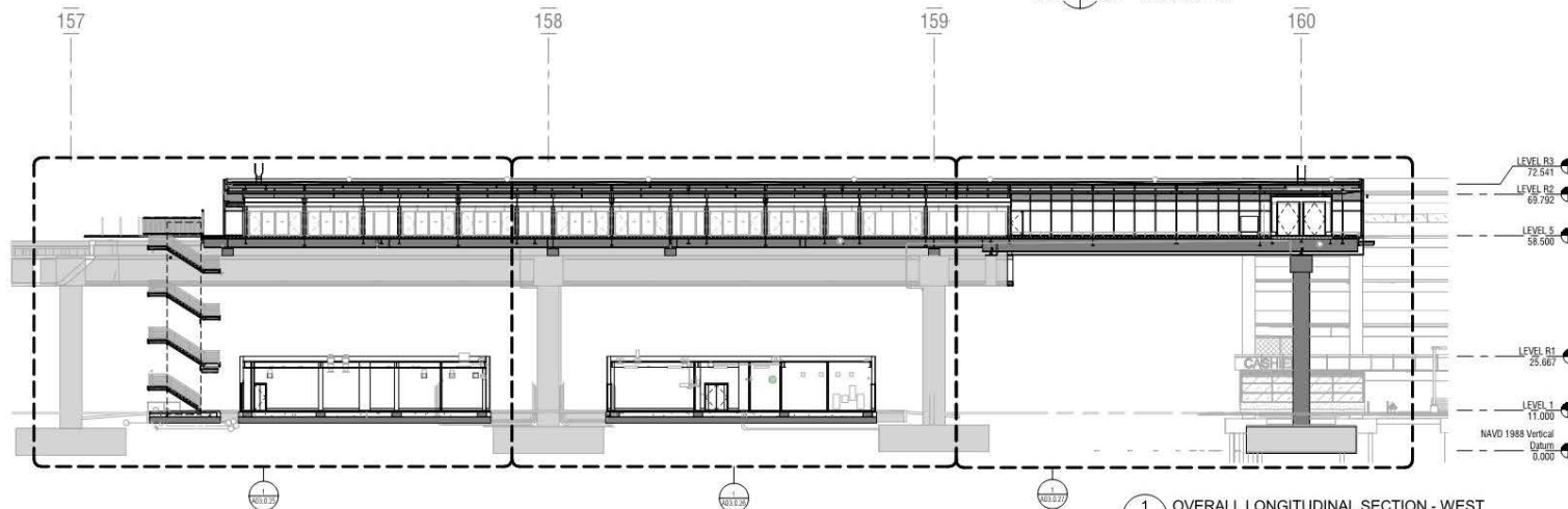
1 OVERALL LONGITUDINAL SECTION - WEST A02.5.01 | A03.0.21 SCALE: 1/16" = 1'-0"
