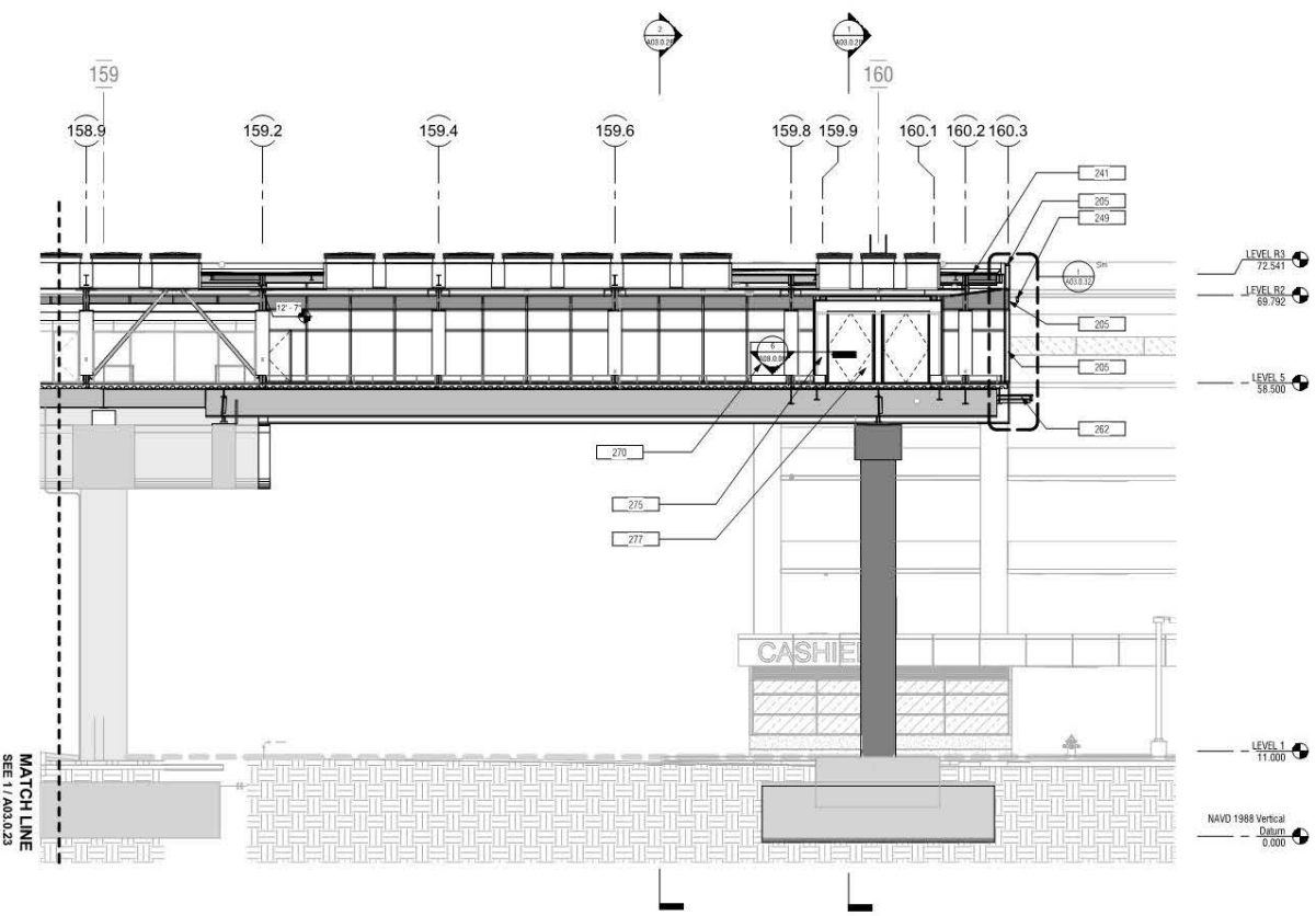
1 LONGITUDINAL SECTION - CENTERLINE SECTOR 3 OF 3 A03.0.21 | A03.0.24 SCALE: 1/8" = 1'-0"
