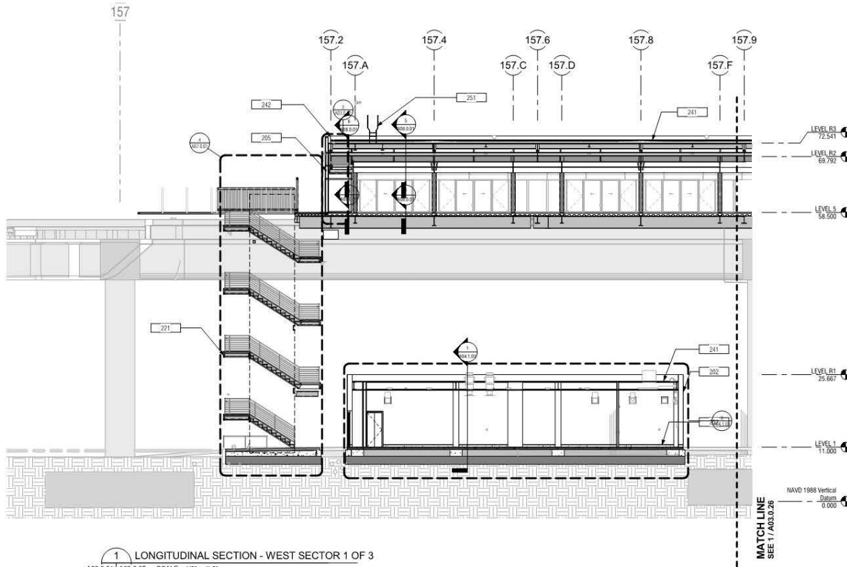
1 LONGITUDINAL SECTION - WEST SECTOR 1 OF 3 A03.0.21 | A03.0.25 SCALE: 1/8" = 1'-0"
