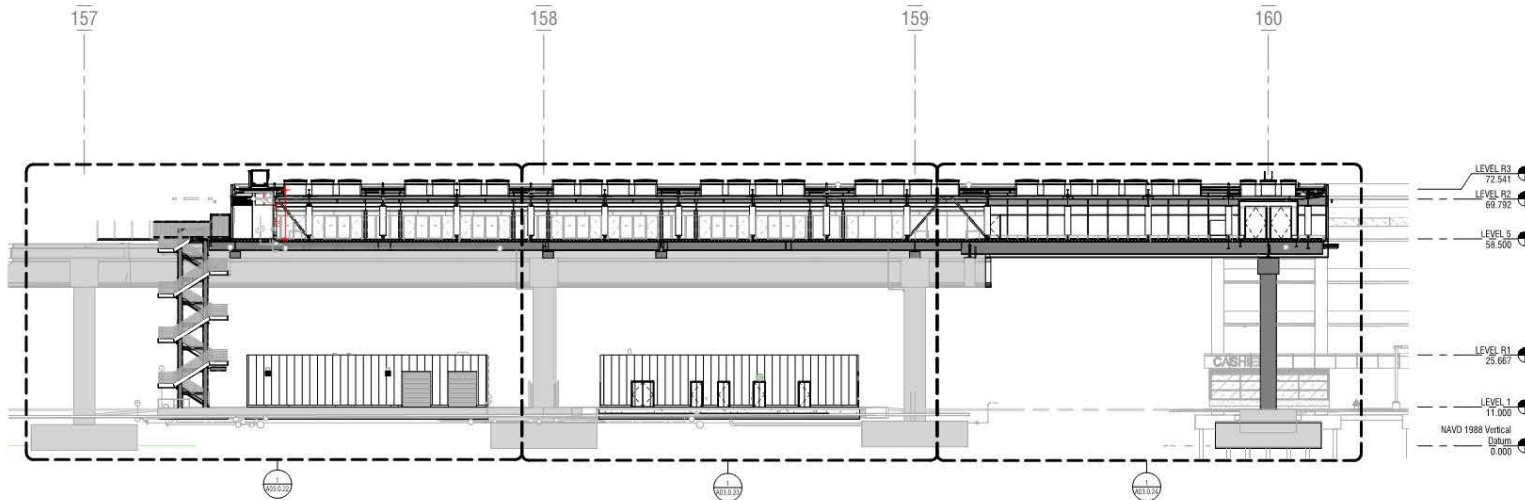
2 OVERALL LONGITUDINAL SECTION - CENTERLINE A02.5.01 | A03.0.21 SCALE: 1/16" = 1'-0"
