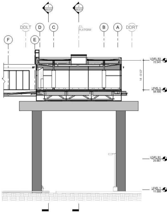
2 TRANSVERSE SECTION - C A02.5.03 | A03.0.28 SCALE: 1/8" = 1'-0"
