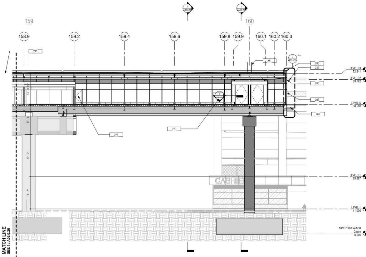
1 LONGITUDINAL SECTION - WEST SECTOR 3 OF 3 A03.0.21 A03.0.27 SCALE: 1/8" = 1'-0"
