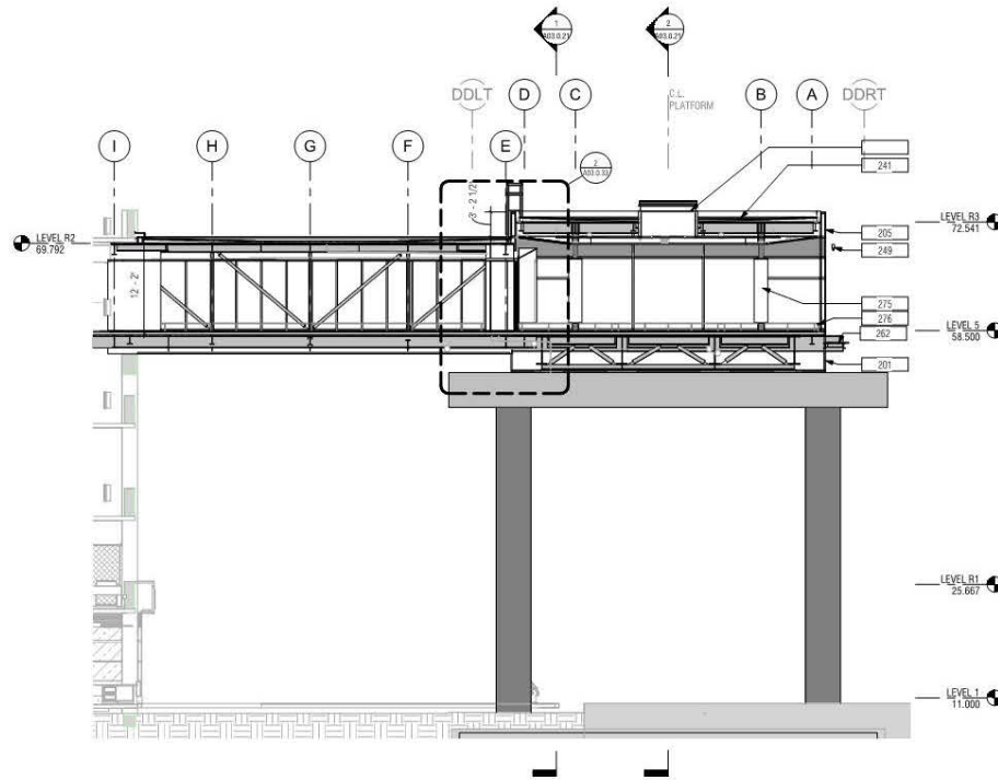
1 TRANSVERSE SECTION - D A02.5.03 | A03.0.28 SCALE: 1/8" = 1'-0"
