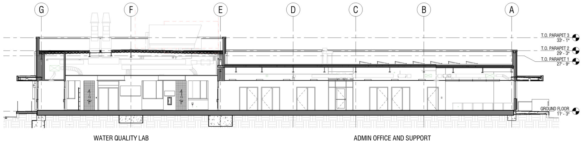
LONGITUDINAL SECTION
