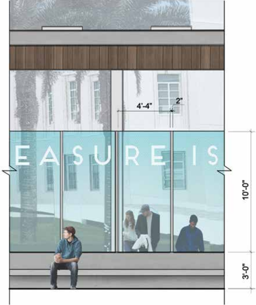
ELEVATION
